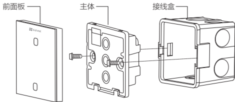
安装示意图
